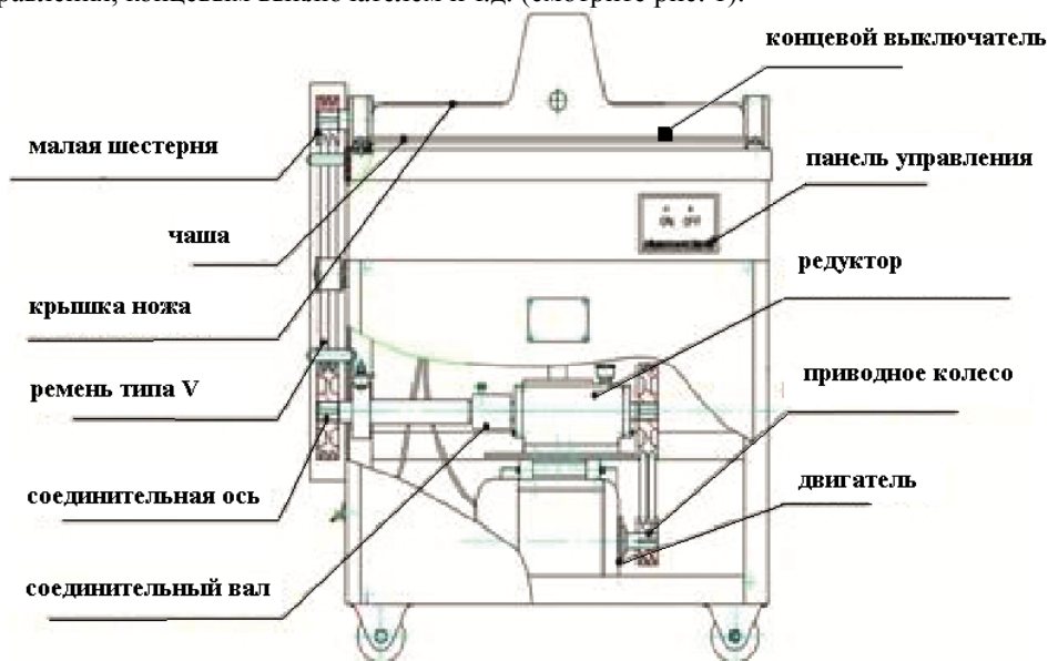
Рис. 1 Основные механизмы оборудования
